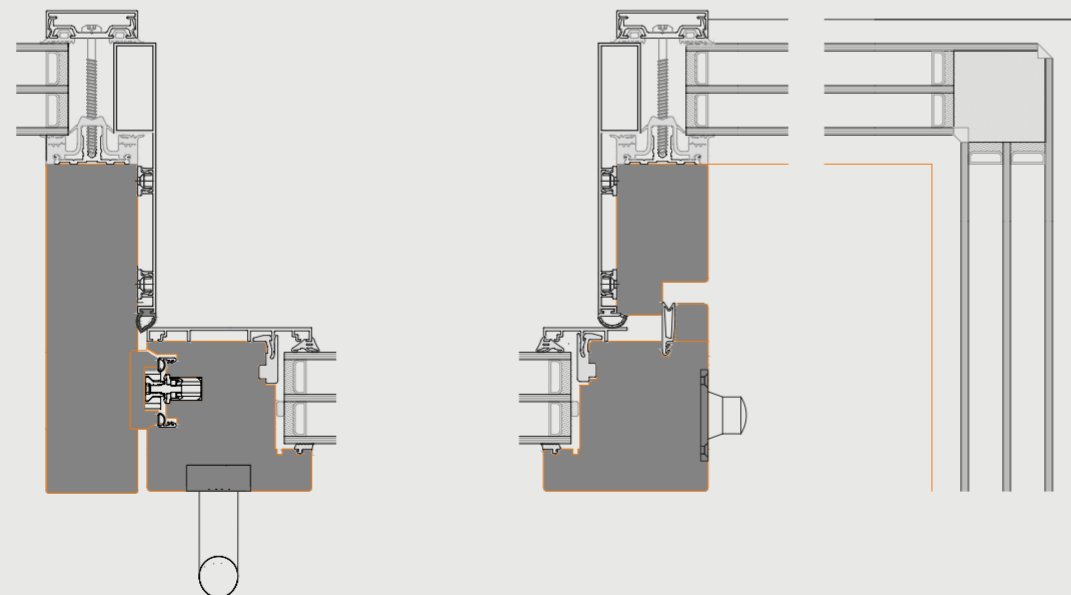
ausführung ganzglasecke
