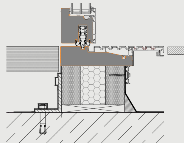
ausführung barrierefrei
